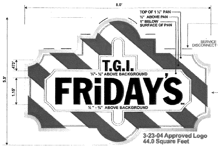
WALL SIGN ELEVATION SCALE: 1/2" = 1'-0"
